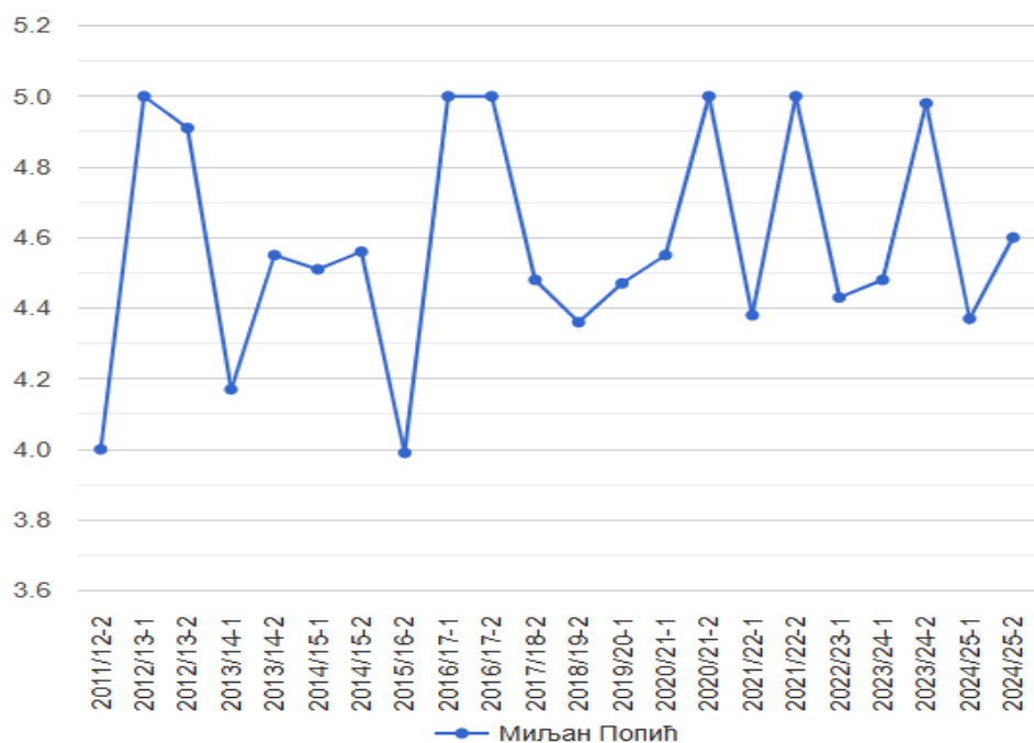
Тренд просјечних оцјена на свим предметима
